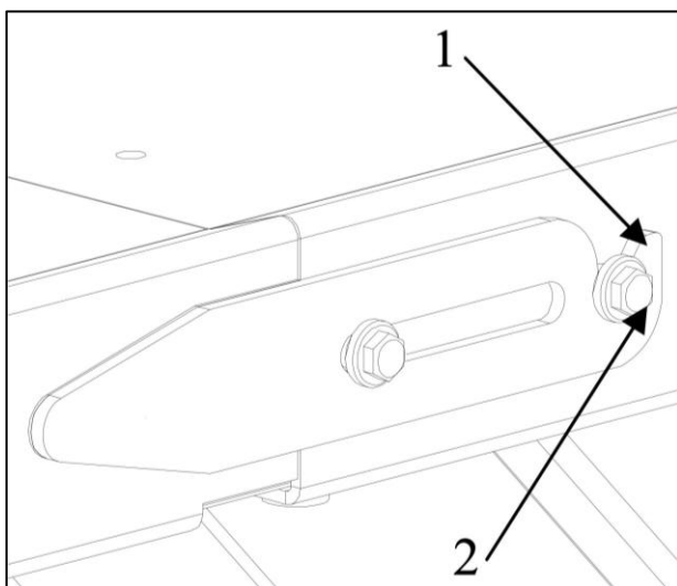
Fig. 7 - Fastgørelse af plade på platformen
