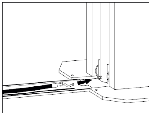
Fig. 17 - Förling av ledning i överkörningsramp
