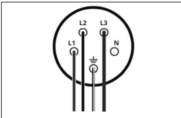
Fig. 7 - Tilslutning af 400V. Monteres der LED-lys på liften, skal "N" også tilsluttes
