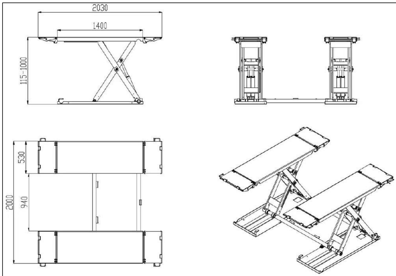
Fig. 3 - Maskinens vägledande mått
