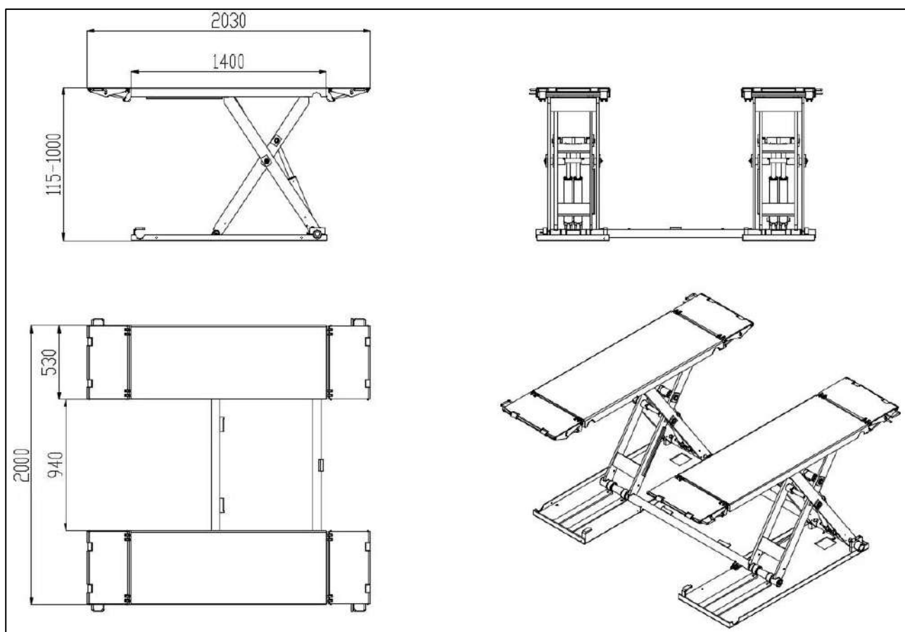
Fig. 3 - Maskinens vejledende mål
