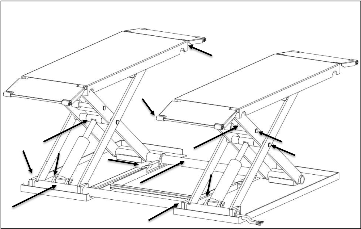
Fig. 9 - Tjek ved årlig vedligeholdelse af maskinen
