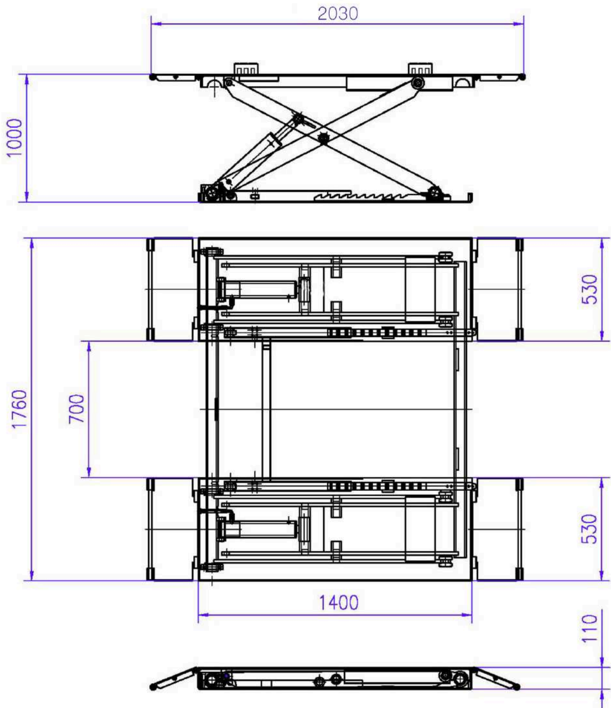
Fig. 3 - Maskinens vejledende mål
