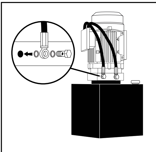
Fig. 5 - Montering af hydraulikslange på motorenhed
