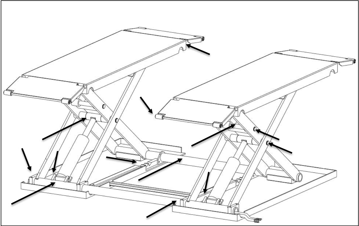
Fig. 9 - Kontrollera vid årligt underhåll av maskinen
