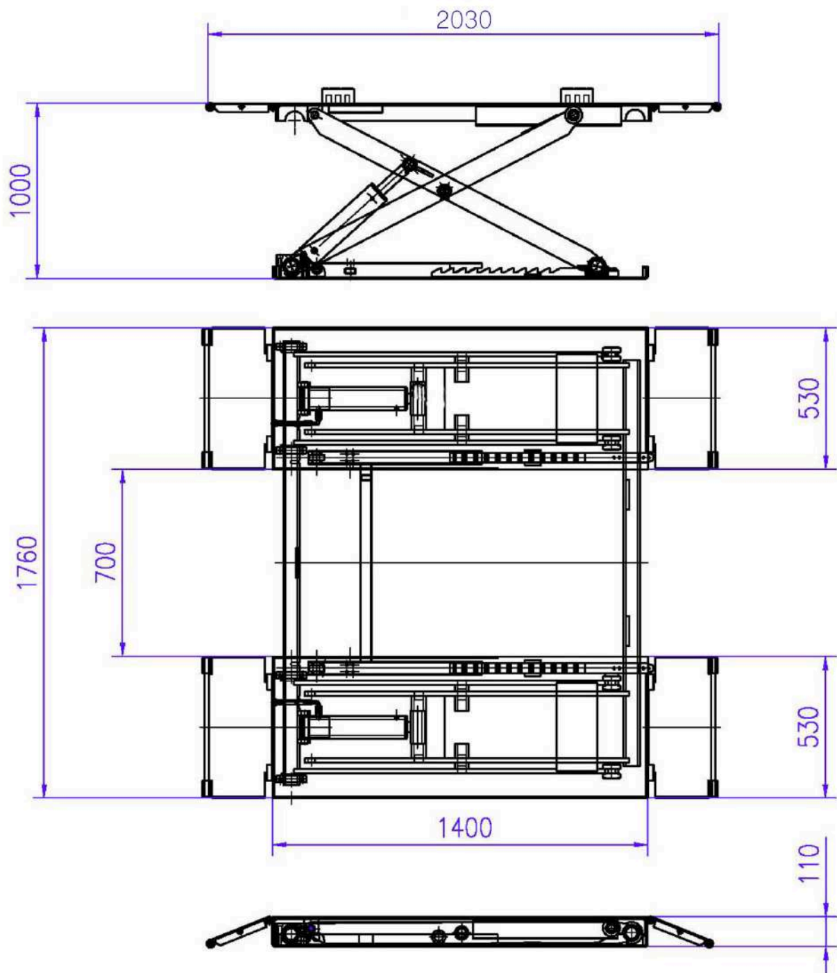
Fig. 3 - Maskinens vägledande mått
