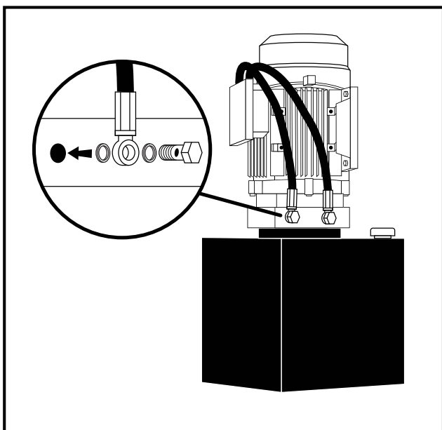
Fig. 5 - Montering av hydraulikslangar på motorenhet
